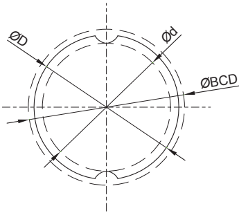
實心花鍵軸
