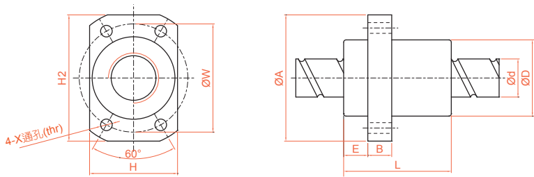
XSY 轉造級系列規格尺寸表
